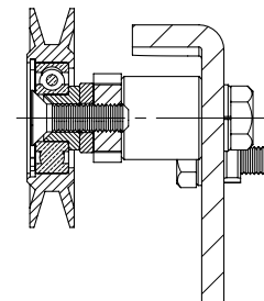
Particolare Fissaggio Puleggia Tendicinghia
